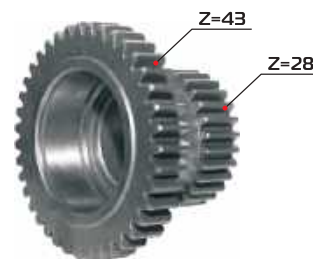
Шестерня 1520-2308062-02
