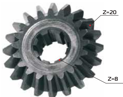
Колесо зубчатое КРН-2.1.03.606 М
