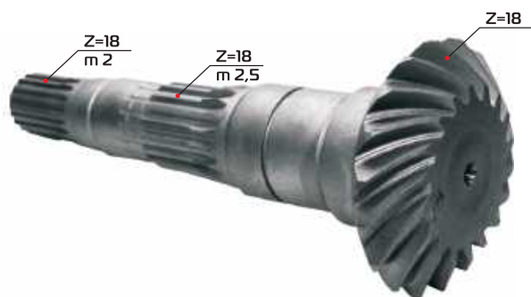
Шестерня РСМ-100.33.03.653
