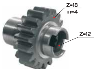
Шестерня 1520-2308061-02
