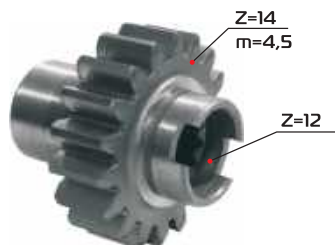
Шестерня 1520-2308061-05
