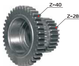
Шестерня 1520-2308062-05
