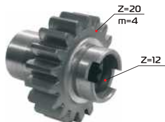
Шестерня 1520-2308061-01
