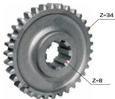
Шестерня скользящая I передачи и заднего хода ЗБ-1701112-А2
